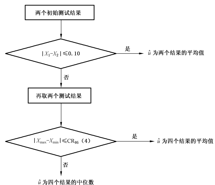
图 H.1 测试结果检查框图
